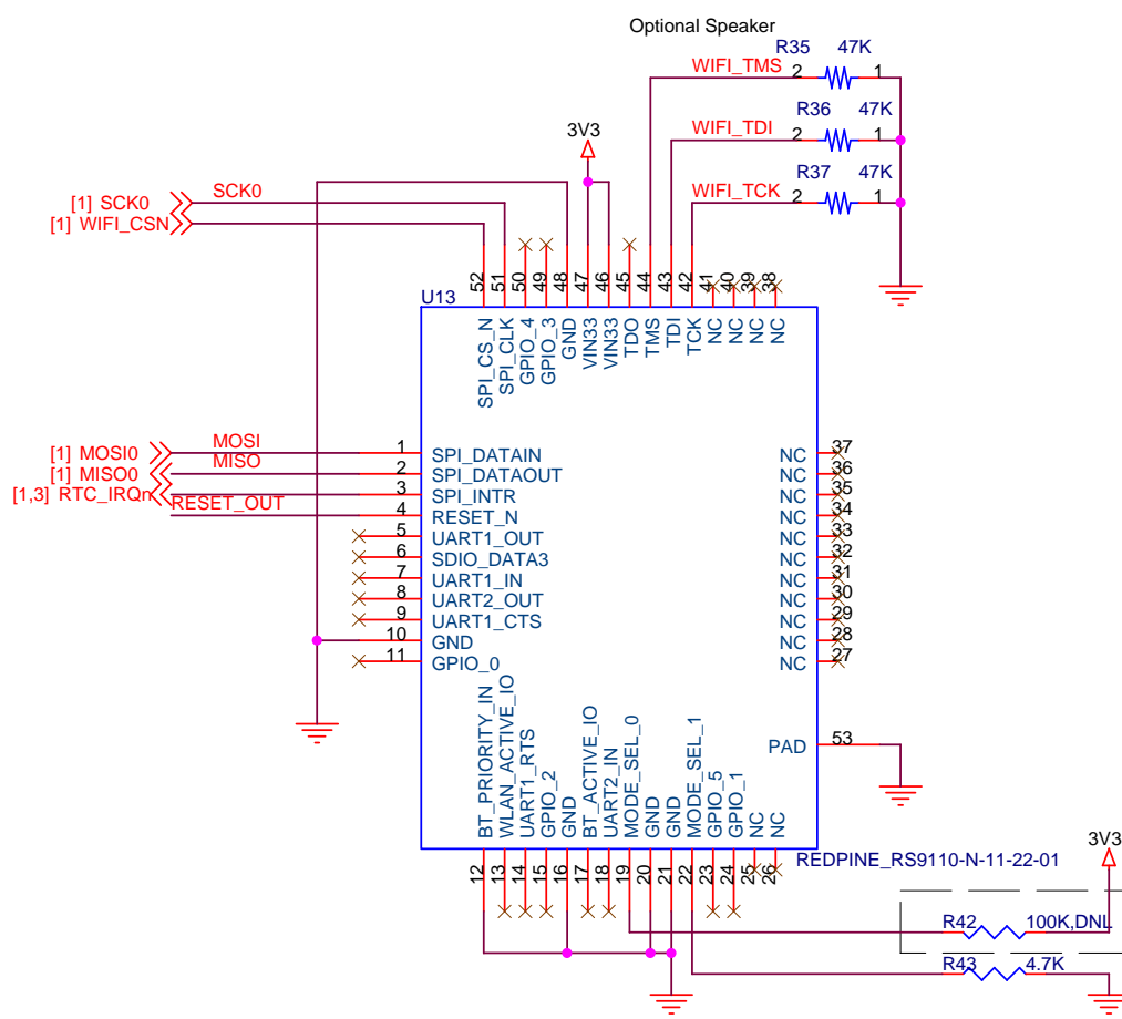
REDPINE WIFI MODULE
